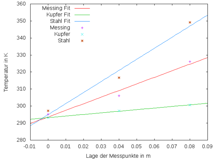
Abbildung 1: Lineare Regression
