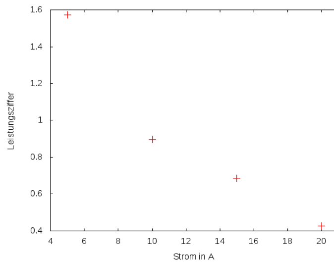
Abbildung 3: Leistungsziffer
